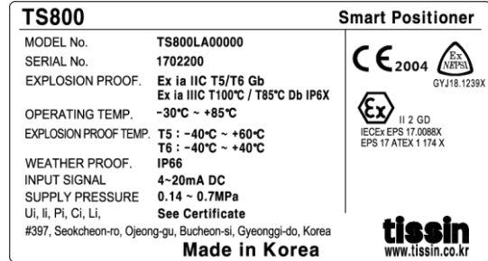
<ATEX 认证名牌>
