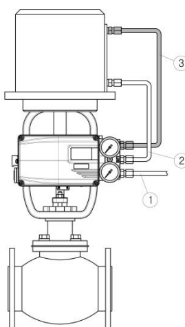
<直行程双作用型>
