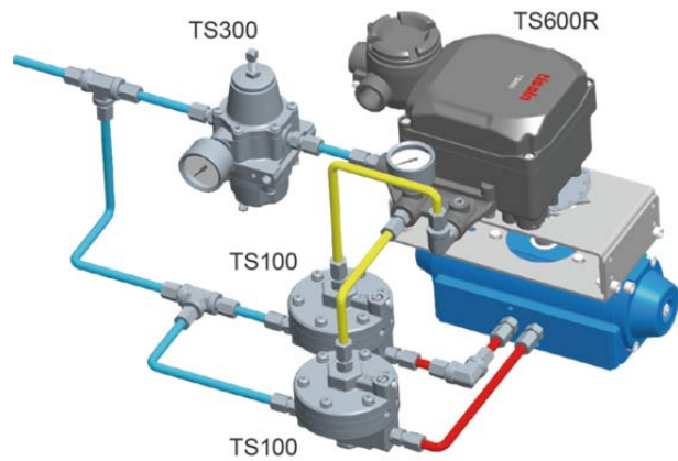
<복동형 액츄에이터 설치 예>
