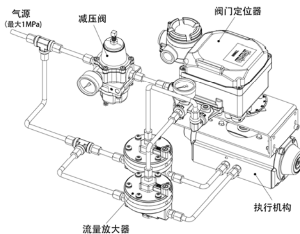
<双作用执行机构安装例图>
